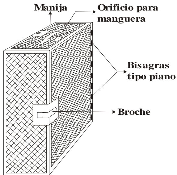
Figura 1. Jaula portátil de Prueba Hidrostática de baja presión útil para proteger al personal de servicio durante dichas operaciones. No es usada para Prueba Hidrostática en cilindros de gas comprimido. No se debe amarrar al piso durante la prueba.
