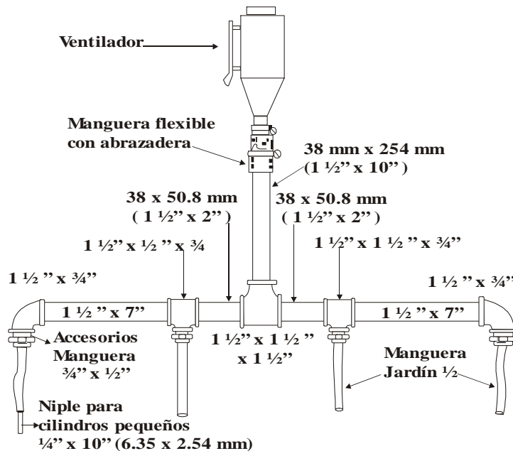
Figura 5 Dispositivo para secar cilindros
